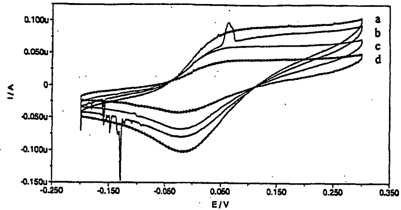
Abbildung 9: CV der TMPD-modifizierten Glukosebiosensoren ohne Schutzschicht, gemessen an unterschiedlichen Tagen, in glukosefreiem PBS-Puffer, (pH 7.4 ; c_{\text{Cl}^-} 154 mM), v = 50 \text{ mV/s} a: 1. Tag ; b: 9. Tag ; c: 18. Tag ; d: 46. Tag
